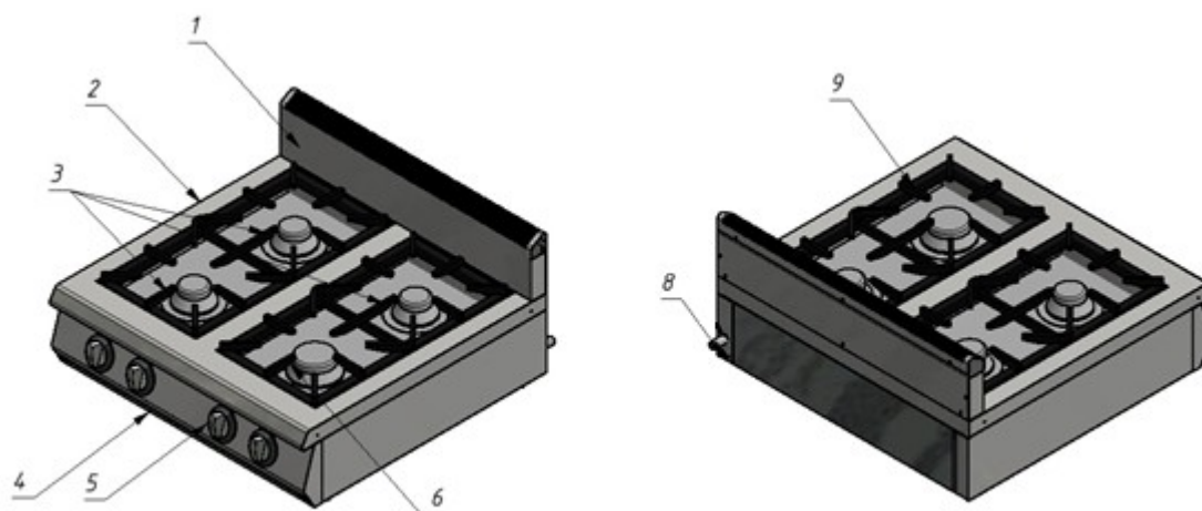
Рисунок 3 – Устройство плиты газовой Ф4ПГ/800
